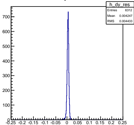
h_dy_res
