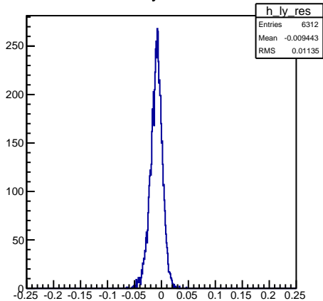
h_ly_res
