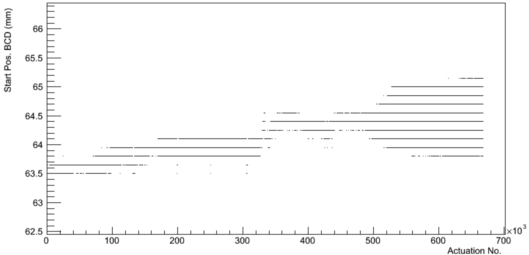
S1.1(R78) - Start Pos. BCD (mm)
